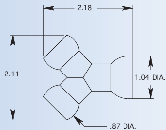
1/2" Y MOLDED
